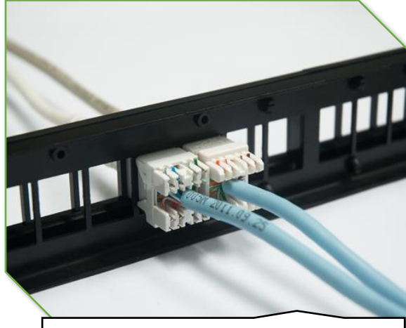
لوحة توصيل بمقاييس (RJ45) قابلة لل فك
