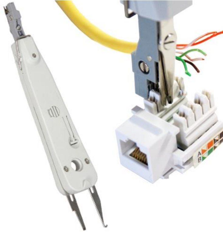
شكل رقم ٦٨: دباسة الأسلاك (Punch Down Tool)
