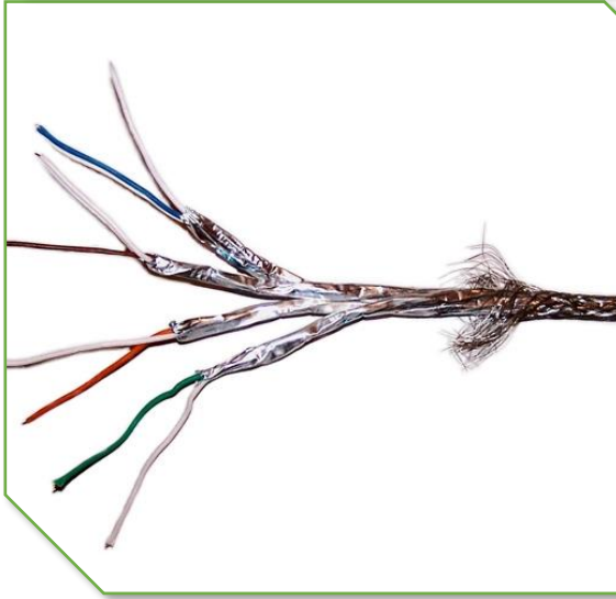
شكل رقم ٣٦: تغليف فردي و عام "S/FTP"
