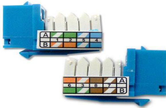
شكل رقم ١٤٠: ترتيب الألوان حسب الترتيب القياسي (EIA/TIA A, B) صورة من الجنب لمقبس RJ45
