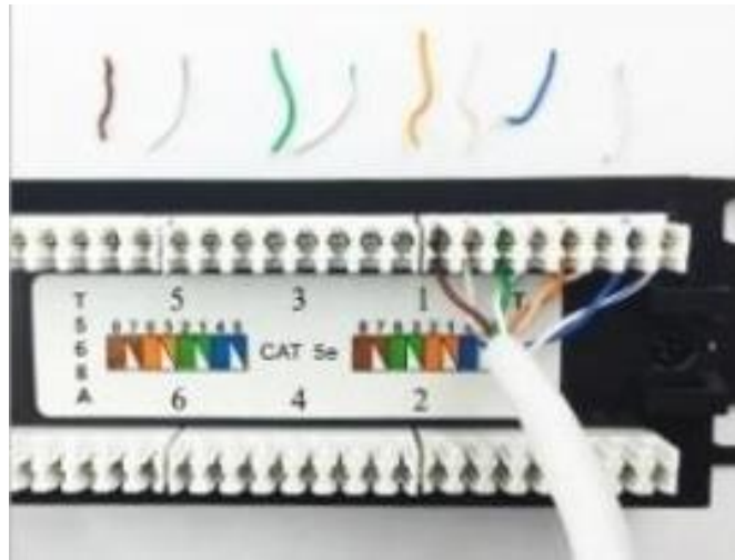
شكل رقم ١٣٣: الشكل النهائي بعد قص أطراف الأسلاك الزائدة
