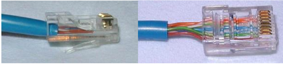
شكل رقم ٨٢: الإدخال الخاطئ لأطراف الكابل في وصلة RJ45
