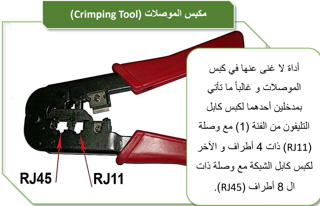
شكل رقم ٢٥: مكبس الموصلات
